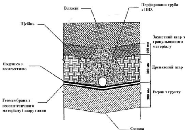
Рис. 3.4. Схема облаштування протифільтраційного екрану в основі полігону (європейська практика)
