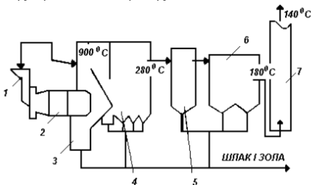
Рис. 2.3. Принцип роботи лінії спалювання:
