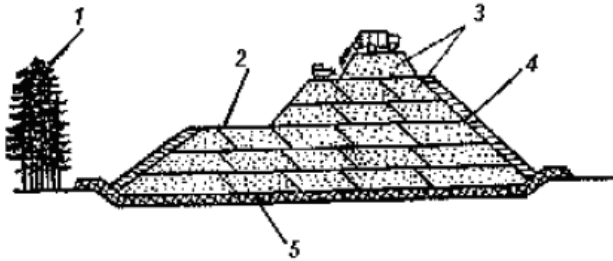
Рис. 3.3. Елементи загальної схеми полігону для твердих відходів: 1 — лісозахисні смуги (зелена зона); 2 — проміжний ізолюючий шар; 3 — відходи; 4 — вкриваючий зовнішній шар рослинного ґрунту; 5 — природна або штучна водотривка основа (глина)
