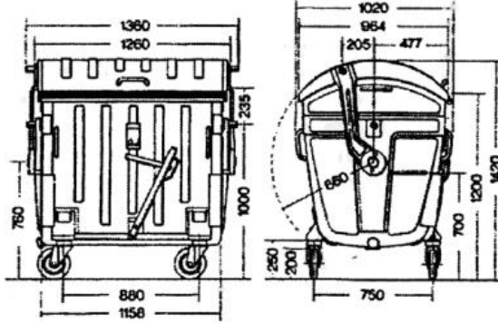
Рис. 3.8. Контейнер для збору ТПВ ємністю 1,1 м 3
