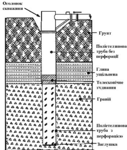
Рис. 3.7. Загальний вигляд свердловини для видобутку біогазу
