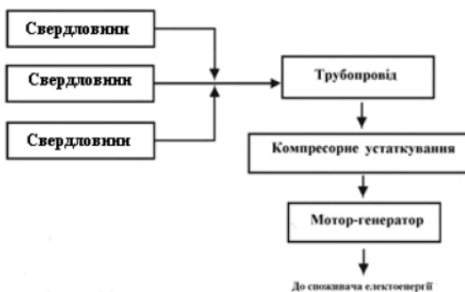
Рис. 3.6. Блок-схема видобутку та утилізації біогазу
