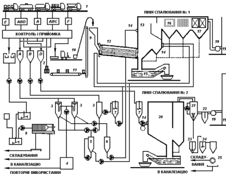
Рис. 2.2. Технологічна схема заводу «Комунікемі»:
