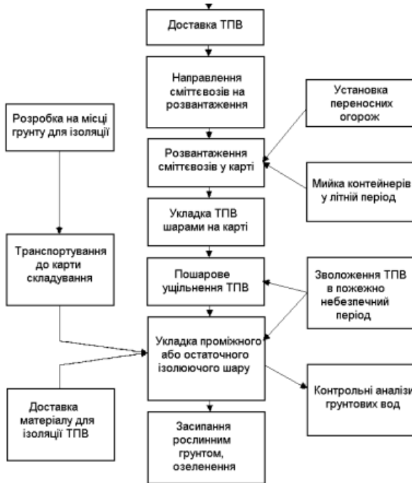
Рис. 3.9. Основні технологічні операції при експлуатації полігонів
