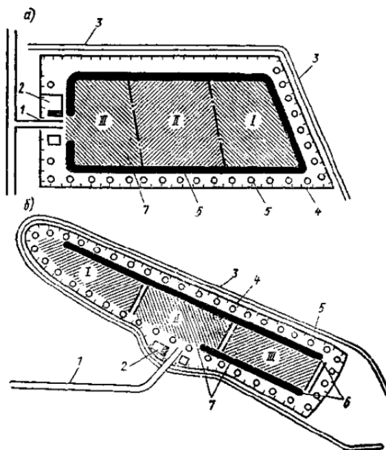
Рис. 3.1. Приклади горизонтального планування полігонів: а) при співвідношенні довжини і ширини менше 1:2; б) при співвідношенні довжини і ширини більше 1:3; 1 — під'їзна дорога; 2 — господарська зона; 3 — канава з насипним валом; 4 — загорожа; 5 — зелена зона; 6 — ґрунт для ізолюючих шарів; 7 — майданчики складування відходів; I, II і III — черги експлуатації
