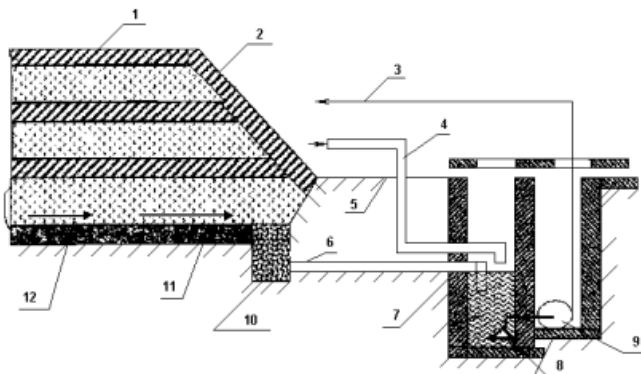
Рис. 3.10. Схема збору дренажних вод та вод від мийки контейнерів:
