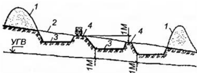
Рис. 3.2. Висотне розміщення котловану в основі полігону: 1 — кавальєр ґрунту; 2 — поверхня ділянки до розробки котловану; 3 — основи ділянок складування; 4 — дорога
