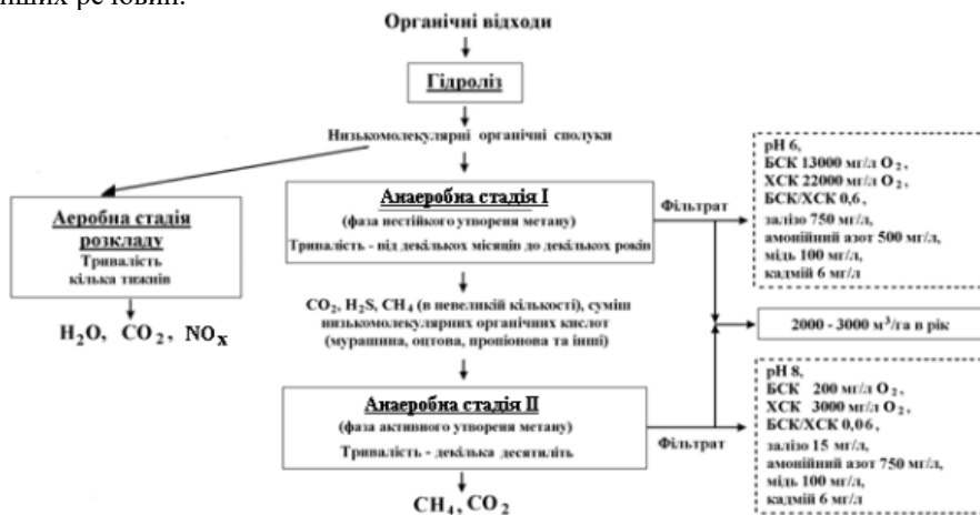
Рис. 3.5. Принципові процеси розкладу органічних сполук при полігонному захороненню ТПВ (основні стадії розкладу, склад утворених продуктів і фільтрату)
