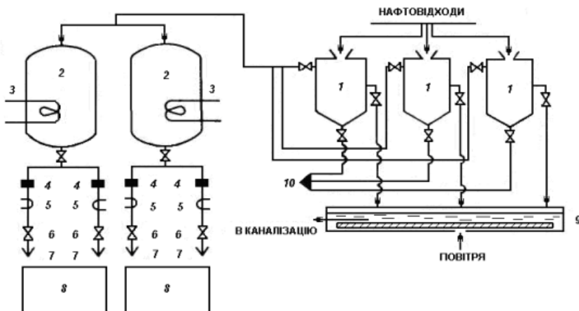
Рис. 2.1. Схема спалювання нафтовідходів на заводі «Мілан-2»:
