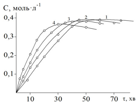
Рис. 3. Вплив температури на кінетику накопичення ацетофенону при окисненні метилфенілкарбінолу озоноповітряною сумішшю в ацетатній кислоті. [O_3]_0 = 5,2 \cdot 10^{-4} , [ArH]_0 = 0,4 моль·л -1 , \omega = 30 л·год -1 , V_p = 10 мл. Температура: 15 (1), 20 (2), 30 (3), 40 (4) ° С
