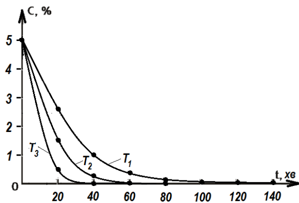
Рис. 2. Залежність концентрації СІМАЗИН від часу переробки: 1 – температура 200 °С; 2 – температуру 250 °С; 3 – температура 300 °С
