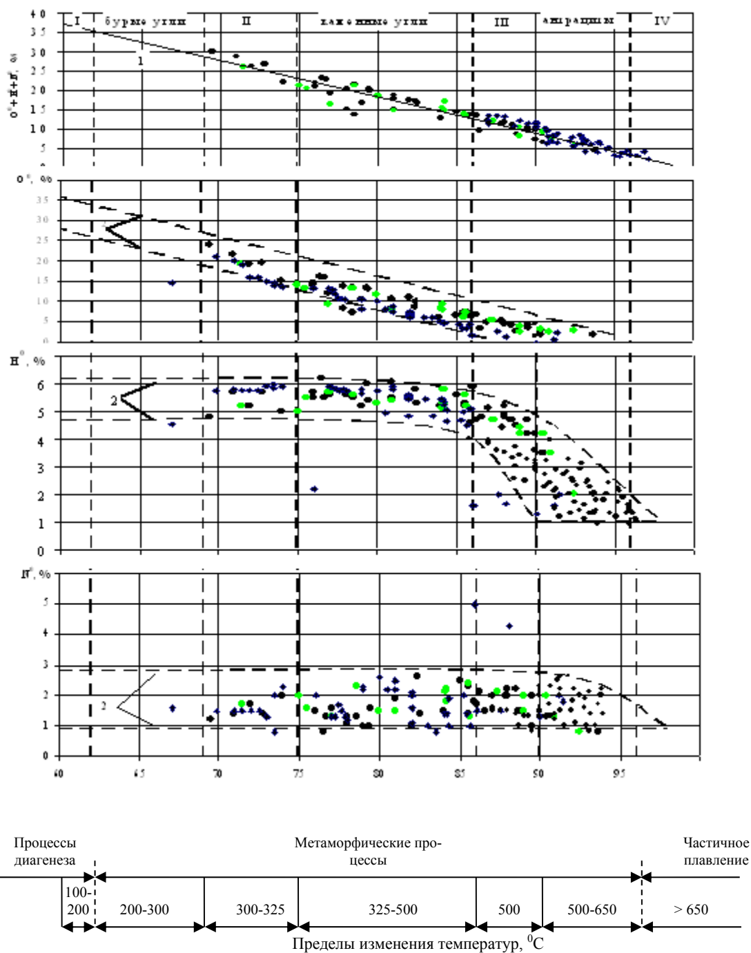
Рис. 1. Залежність зміни вмісту вуглецю з сумарним вмістом O°, H° і N° (а), O° (б), H° (в) і N° (г): I, II, III, IV - орієнтовні діапазони температури і вмісту C°, в яких змінюються властивості при переході відповідно від торфу до бурого вугілля, від бурого до кам'яного, від кам'яного до антрациту, від антрациту до графіту;
