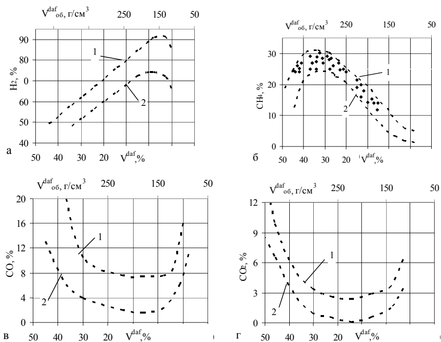
Рис. 4. Залежності змісту газів термічного розкладання вугілля від вагового ( V^{daf} ) і об'ємного ( V^{daf}_{об} ) виходу летючих речовин: 1,2 – верхня та нижня межі зміни параметрів [6] • – експериментальні дані [6]
