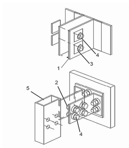
Рис. 6. Вузли кріплення стійок навісних вітражів: а – за допомогою кронштейна-деталі; б – зі збірним кронштейном; 1 – кронштейн; 2 – втулка; 3 – накладка; 4 – болт з гайкою і шайбою; 5 – стійка
